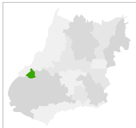
Figura 254. Registro de Lithobates palmipes .
