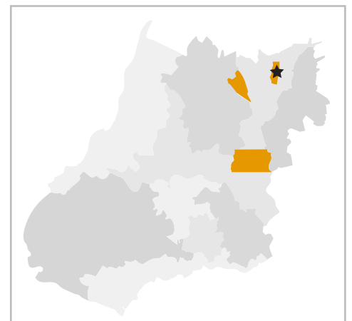
Figura 150. Registros de Adenomera juikitam . Estrela = Localidade-tipo.
