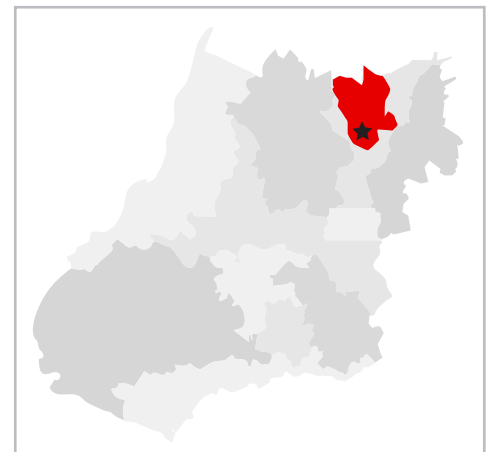
Figura 138. Registros de Scinax rupestris . Estrela = Localidade-tipo.
