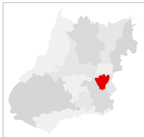
Figura 38. Registro de Vitreorana sp.
