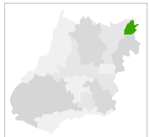
Figura 199. Registros de Pleurodema diplolister .
