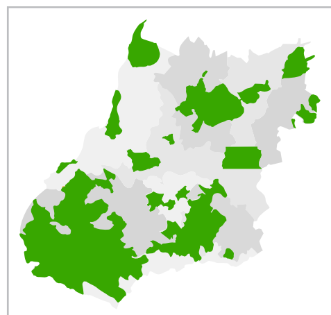
Figura 191. Registros de Physalaemus centralis .
