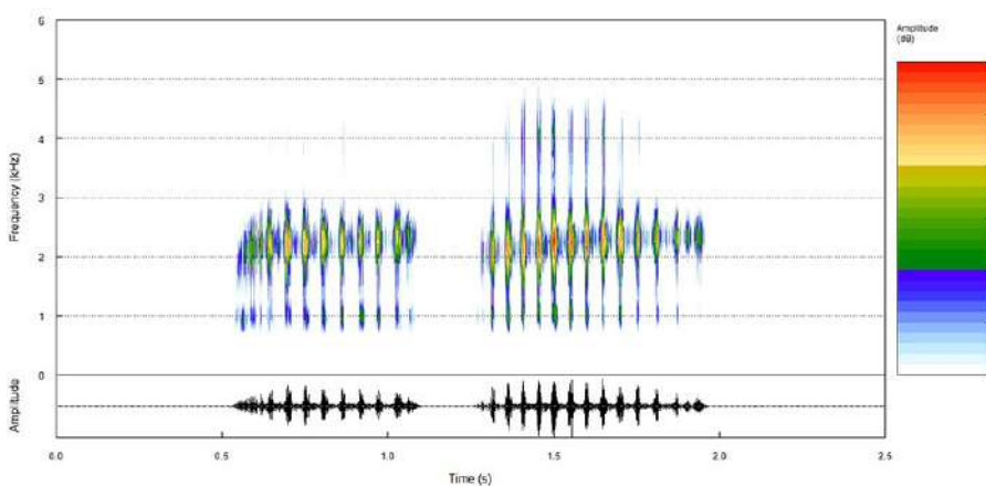
Figura 54. Canto de anúncio de Boana albopunctata , município de Caldas Novas, estado de Goiás.
