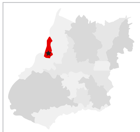
Figura 220. Registro de Chiasmocleis centralis . Estrela = Localidade-tipo.
