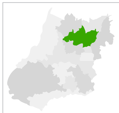
Figura 17. Registros de Rhaebo guttatus .
